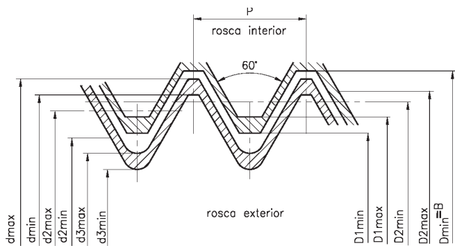
Perfil de base y perfil de los límites
