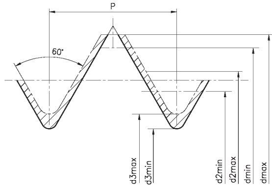
Perfil de base y perfil de los límites
